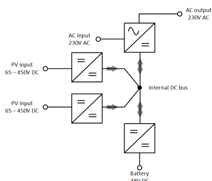
Diagramă bloc Multi RS Solar
